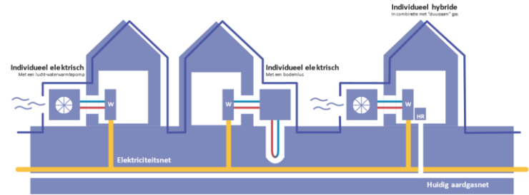
Schematische weergave all-electric en hybride
